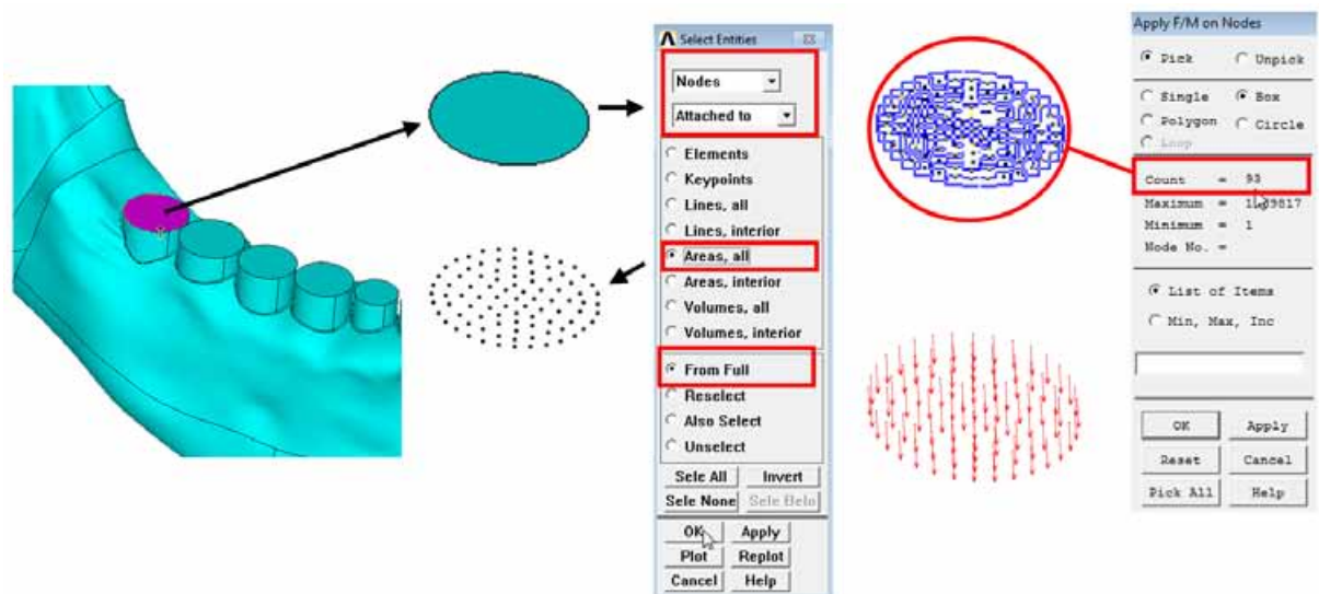
Obr. 5.13 Aplikace síly do uzlových bodů na ploše.
