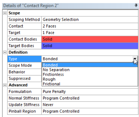
Obr. 5.37 Změna typu kontaktu.
